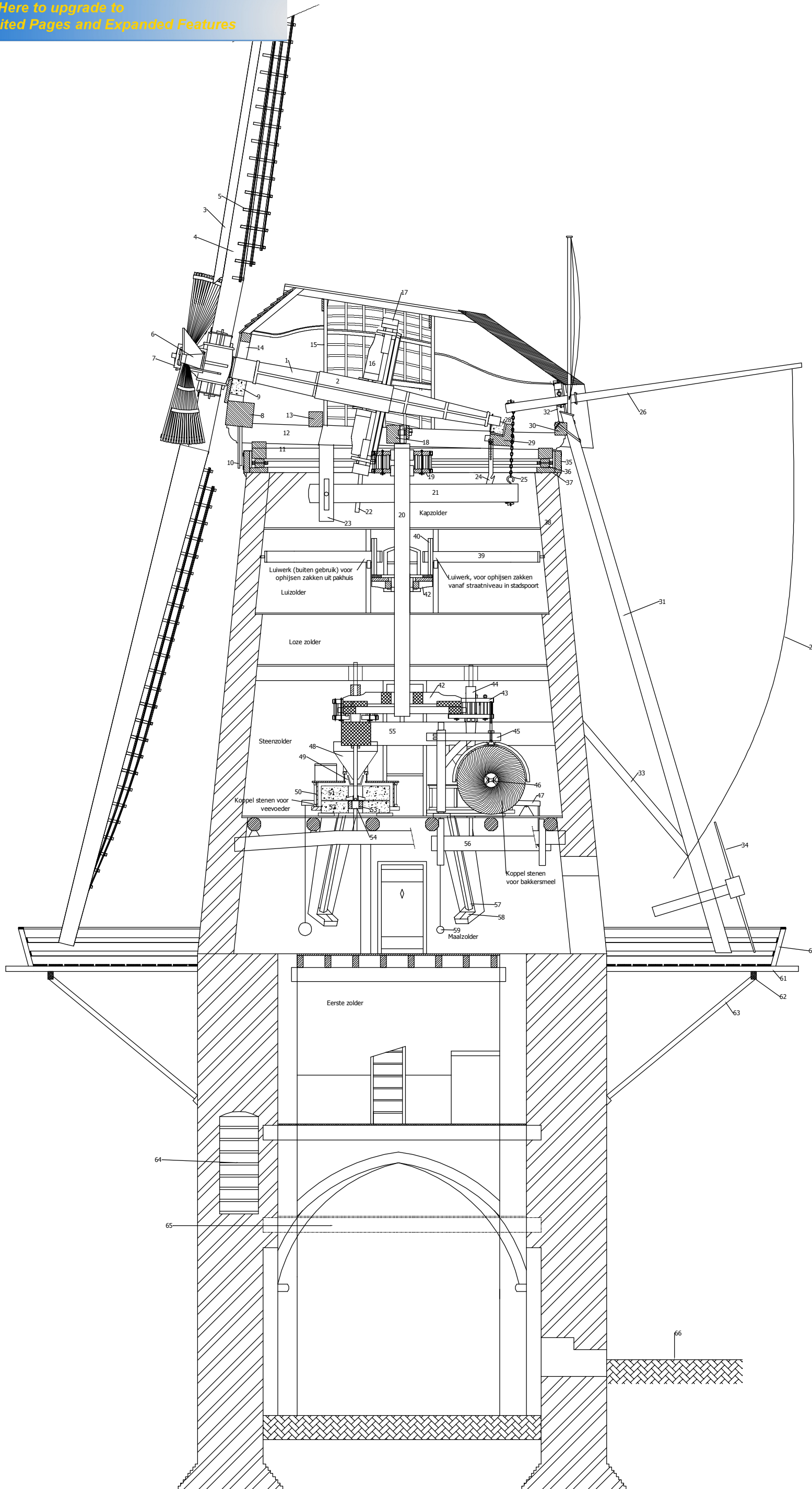
Doorsnede molen gericht naar het noordoosten
